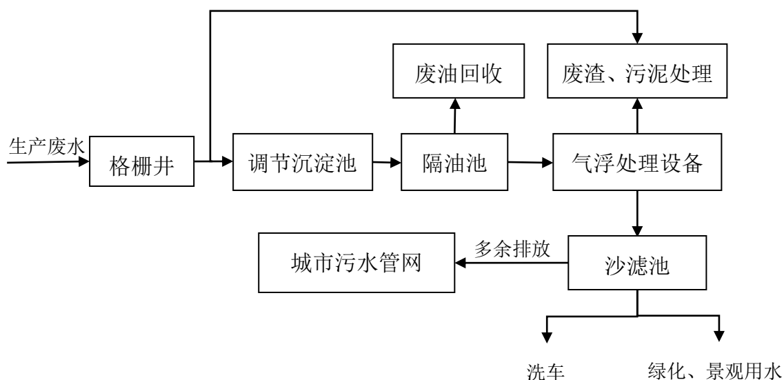
图 7.4.2-2 车辆段、停车场生产废水处理工艺
