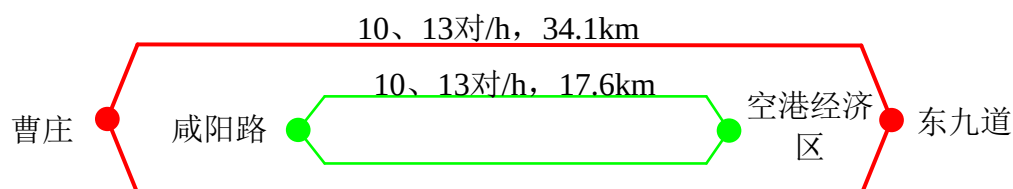
图 3.4-8 M2 线高峰小时列车运行交路
