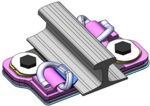
双层非线性减振扣（中等）
