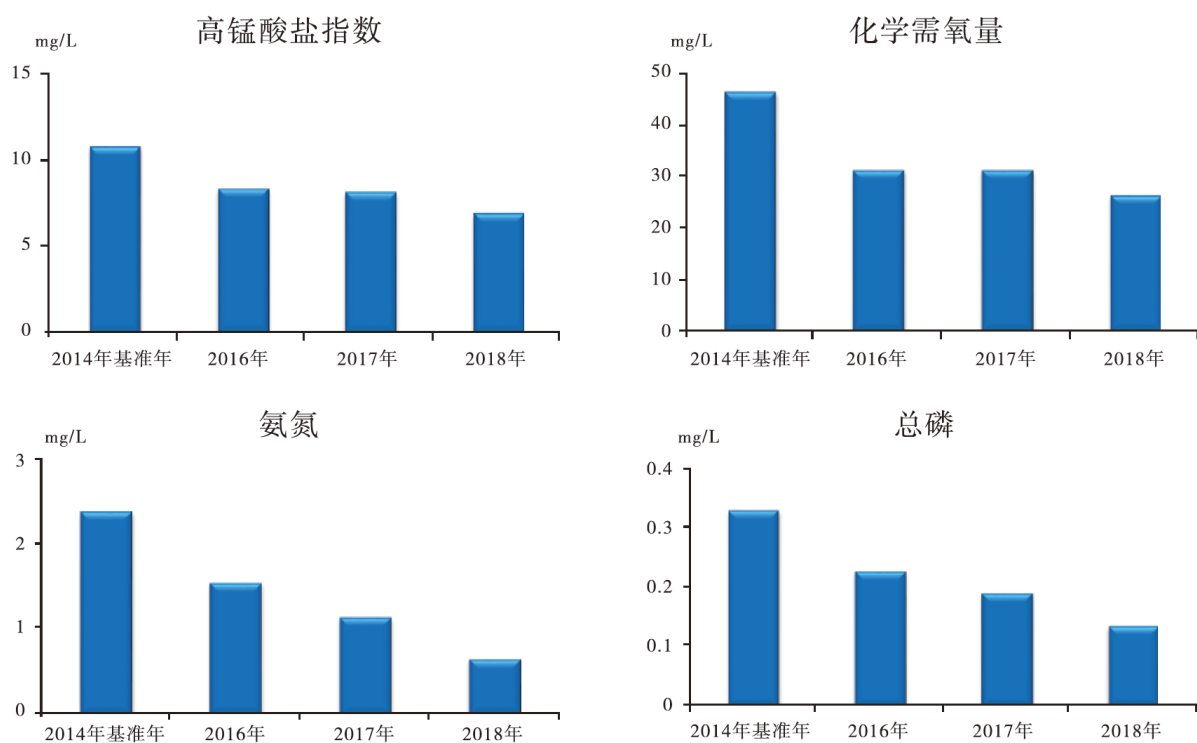
图 4.3-6 主要污染物浓度变化趋势
