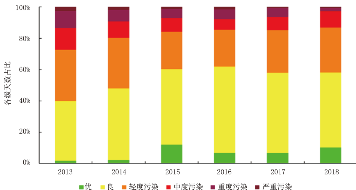
图 4.3-3 环境空气质量级别天数比例
