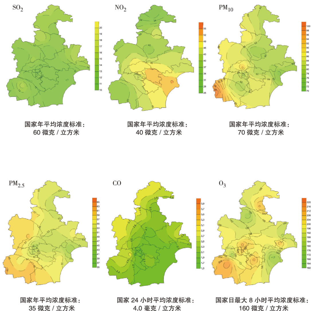
图 4.3-4 天津市环境空气质量空间分布
