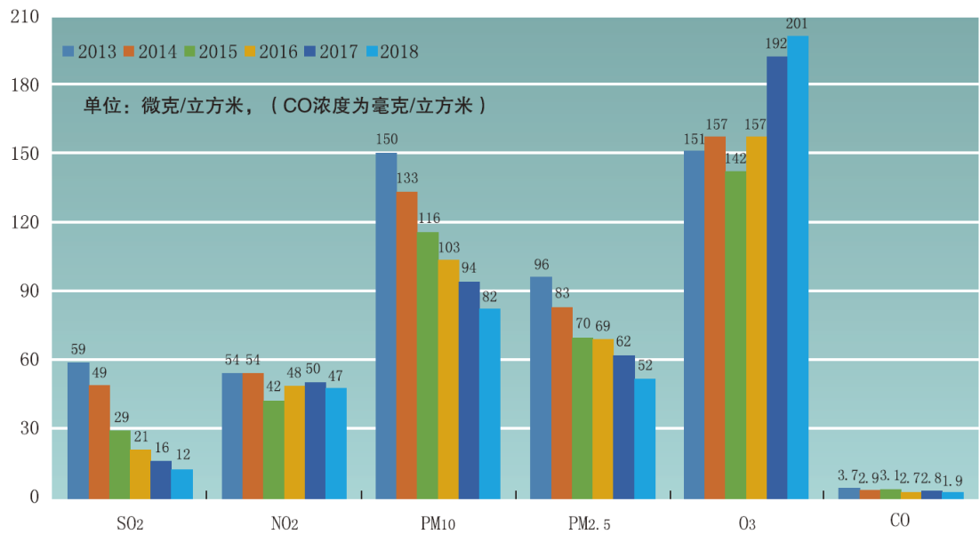
图 4.3-1 2013-2018 年天津市空气中主要污染物年平均浓度值变化趋势
