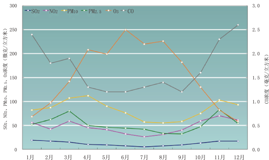
图 4.3-2 六种污染物月变化曲线
