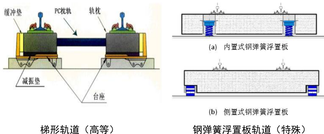
图 9.4-1 几种典型减振措施
