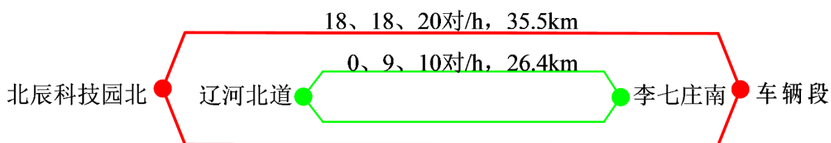
图 3.4-9 M5 线高峰小时列车运行交路图
