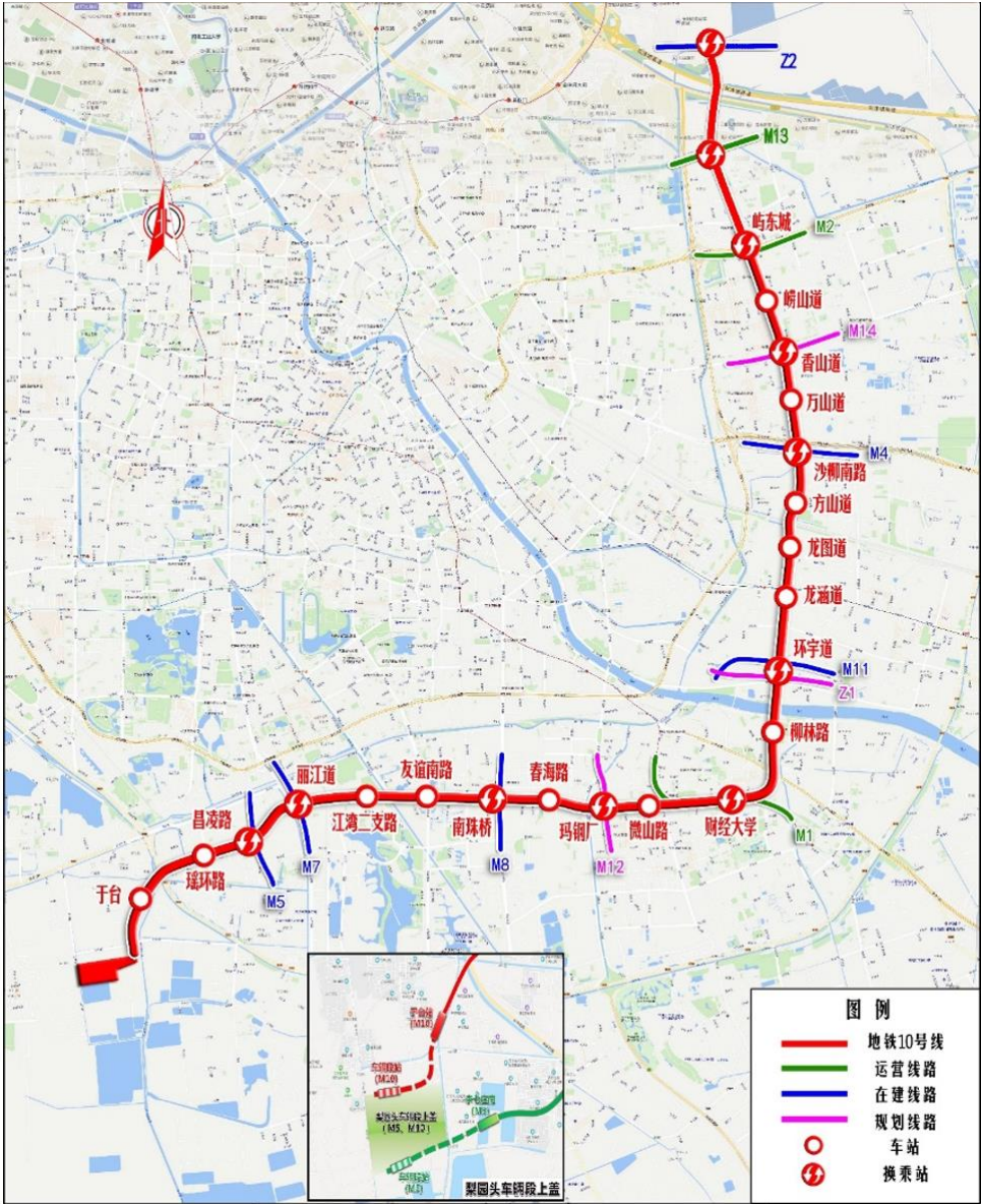
图 3.4-5 M10 延伸梨园头车辆段工程平面示意图
