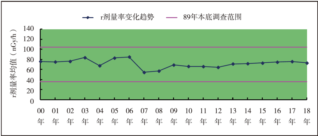
图 4.3-9 2000 年-2018 年辐射环境 \gamma 剂量率变化
